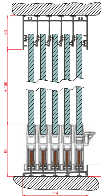
Presjek Sistem sa 5 krila
