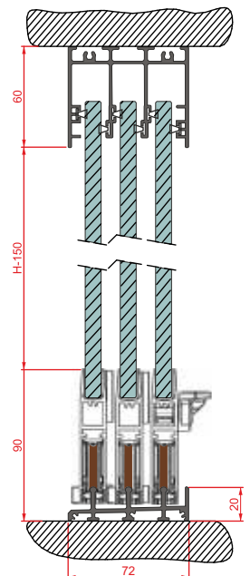
Presjek Sistem sa 3 krila
