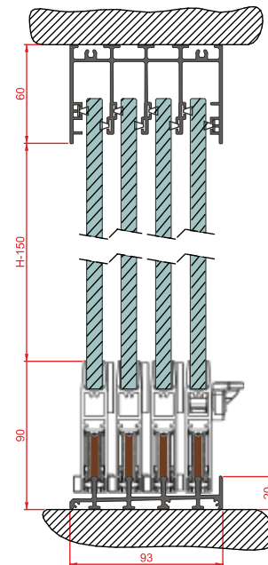
Presjek Sistem sa 4 krila
